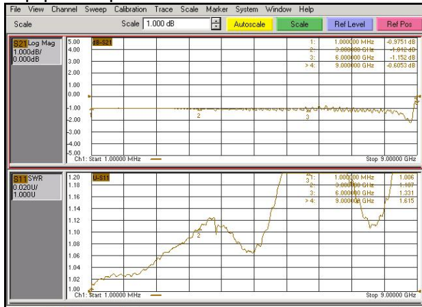
Графики для АЧХ - Log Mag, при отсчётном уровне равном 1 дБ, и для КСВ - SWR
