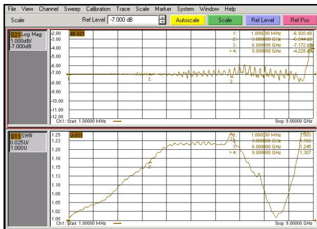
Графики для АЧХ - Log Mag, при отсчётном уровне равном -7 дБ, и для КСВ - SWR
