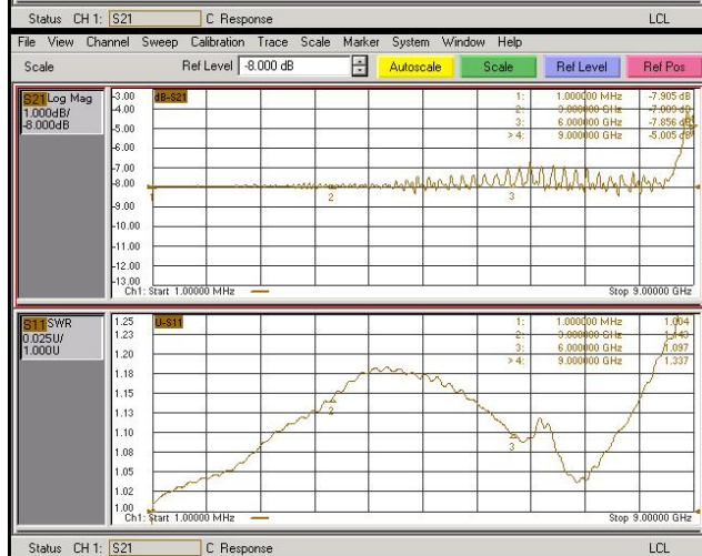
Графики для АЧХ - Log Mag, при отсчётном уровне равном -8 дБ, и для КСВ - SWR
