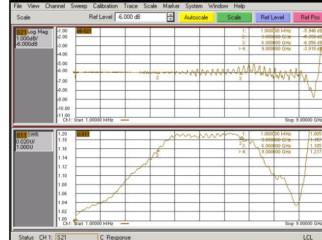
Графики для АЧХ - Log Mag, при отсчётном уровне равном -6 дБ, и для КСВ - SWR
