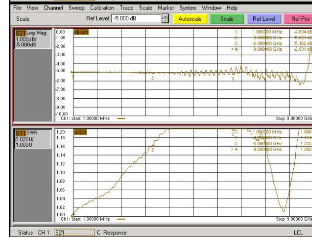
Графики для АЧХ - Log Mag, при отсчётном уровне равном -5 дБ, и для КСВ - SWR
