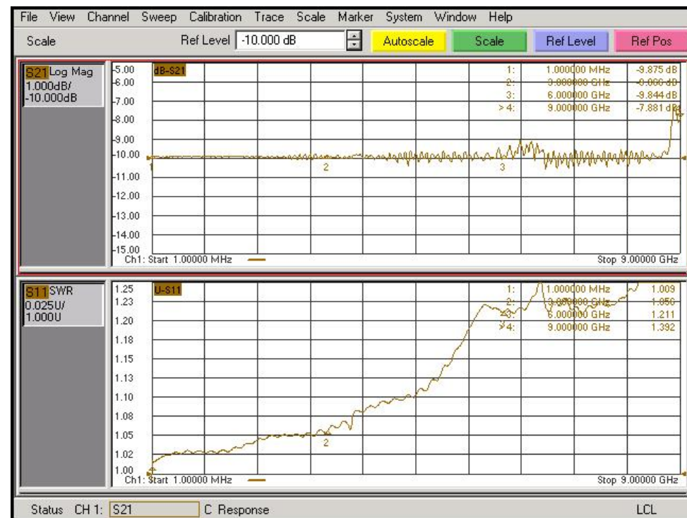
Графики для АЧХ - Log Mag, при отсчётном уровне равном -10 дБ, и для КСВ - SWR
