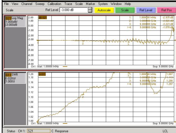
Графики для АЧХ - Log Mag, при отсчётном уровне равном -3 дБ, и для КСВ - SWR
