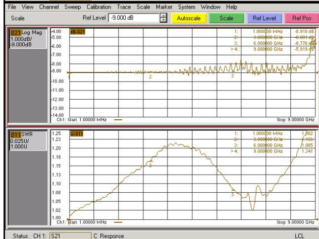
Графики для АЧХ - Log Mag, при отсчётном уровне равном -9 дБ, и для КСВ - SWR
