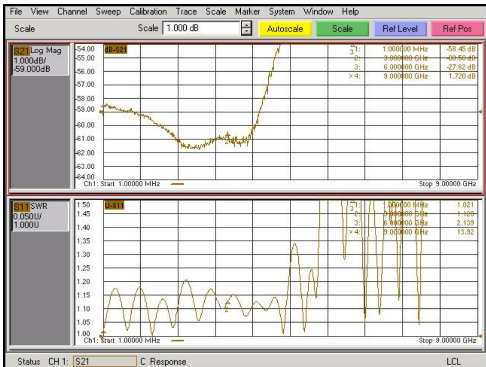
Графики для АЧХ - Log Mag, при отсчётном уровне равном -59 дБ, и для КСВ – SWR
