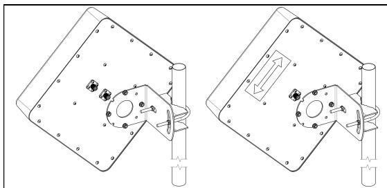
Рисунок 3 – X-поляризация
