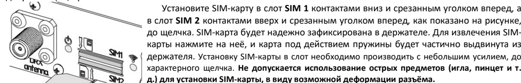
Установка SIM-карт
