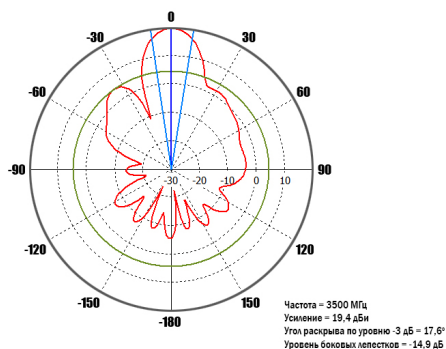
3500 МГц Вертикальная плоскость
